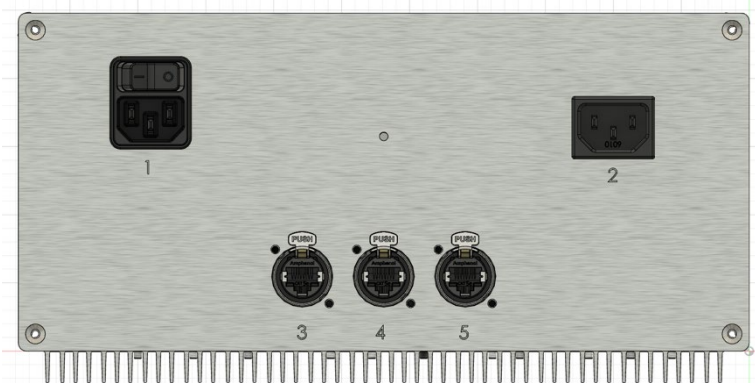
Abb. 2: Anschlussübersicht
