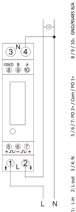
Abb. 7: Anschluss des Energiezählers SDM120
