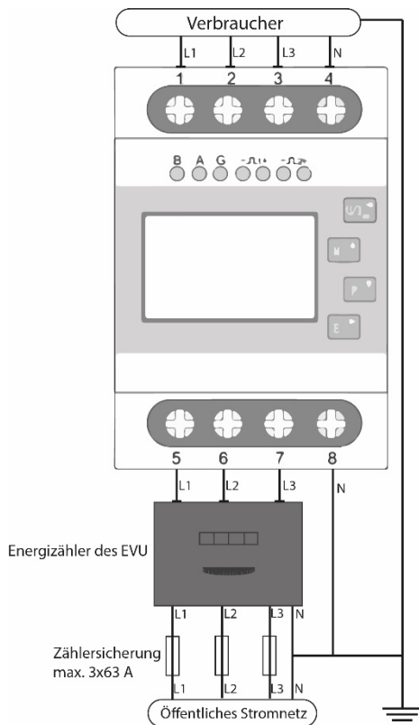
Abb. 6: Anschluss der Leistungsmesser SDM630
