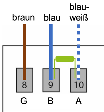
Abb. 10: Installation der Modbusleitung am SDM120
