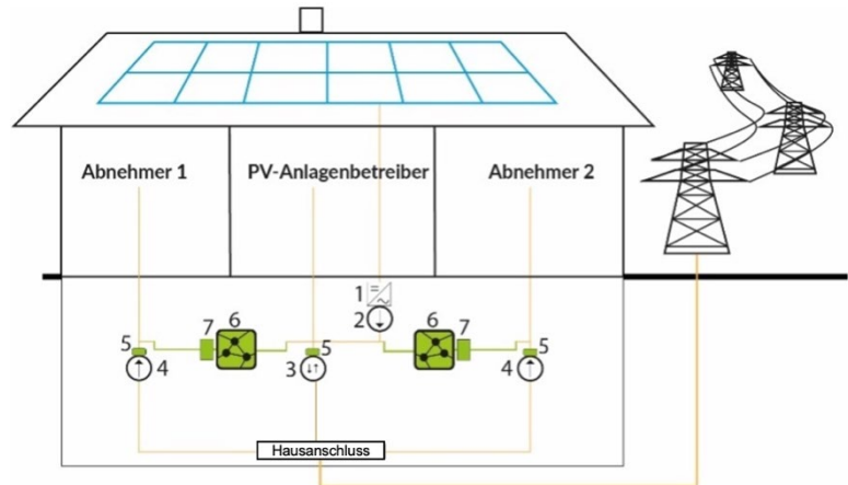
Abb. 1: Schematische Darstellung der Installationsorte bei Versorgung von zwei Abnehmern
