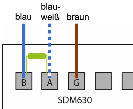
Abb. 9: Installation der Modbusleitung am SDM630 (Abschlusswiderstand beim SDM630 NUR auf Lieferantenseite)
