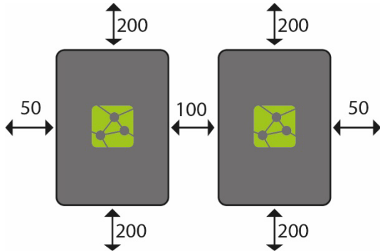
Abb. 4: Wärmeabluft, Angaben in mm
