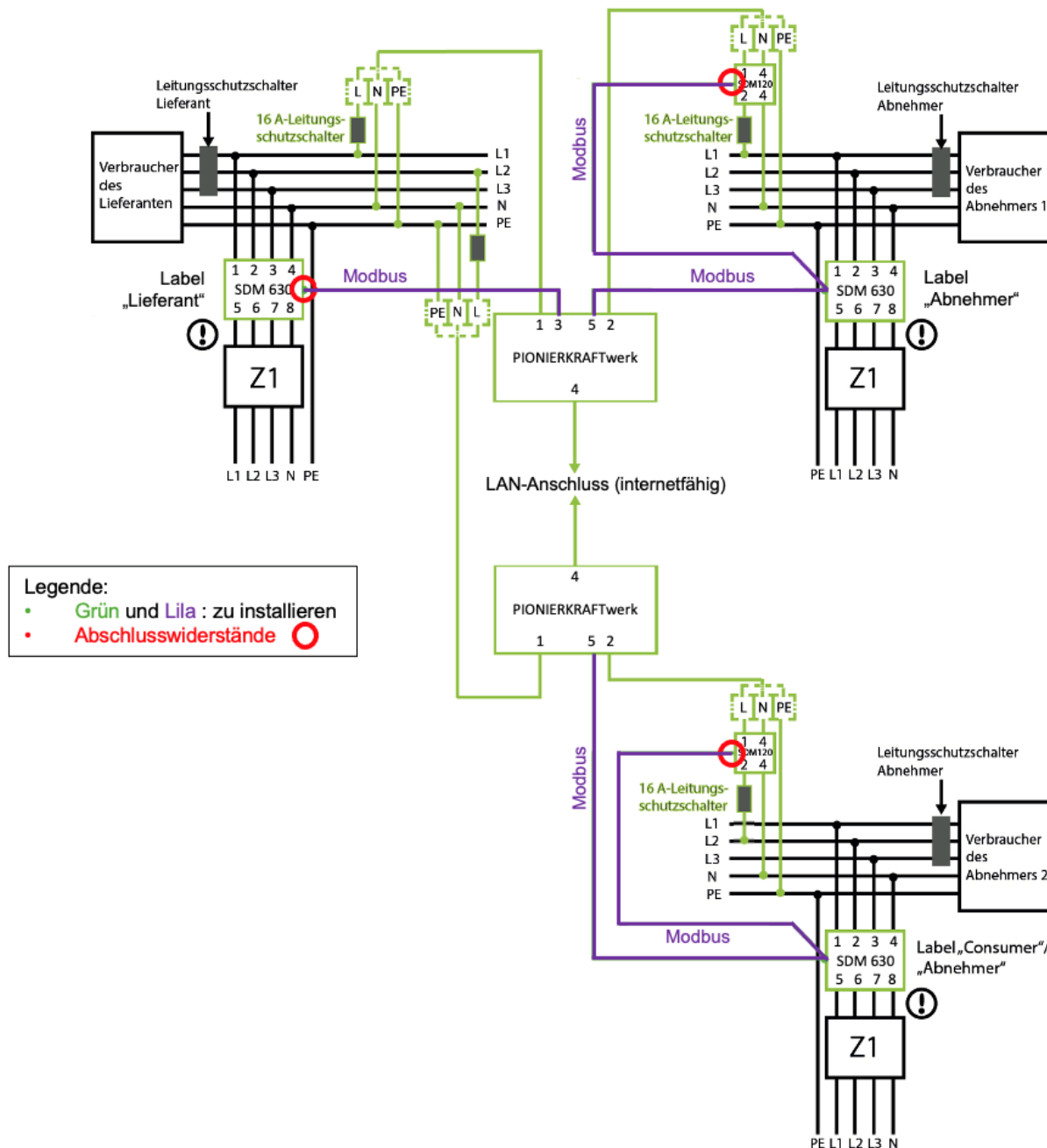
Abb. 5b: Installationsplan bei zwei oder mehreren PIONIERKRAFTwerken
